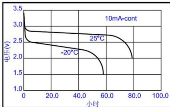
恒流放电曲线
