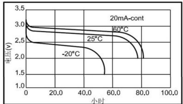
恒流放电曲线
