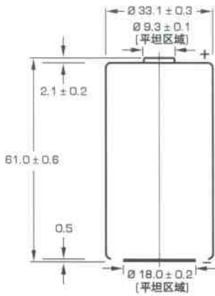
突出正极帽封装形式
