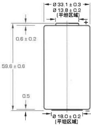
扁平正极帽封装形式
