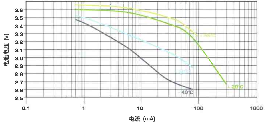
在不同放电电流、温度条件下的平稳电压曲线图 (在放电的稳定阶段)
